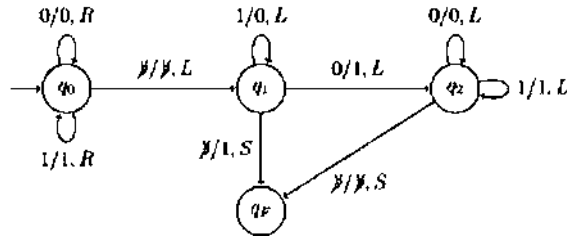
Figura 1. – Una macchina di Turing che calcola il successore di un numero binario.
