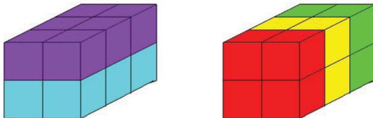
Fig. 1. – Due modi di affettare una matrice 3 \times 2 \times 2
