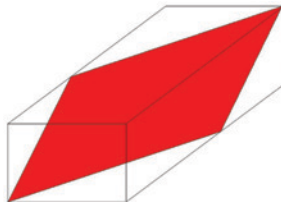
Fig. 8. – La diagonale di una matrice di formato bordo.
