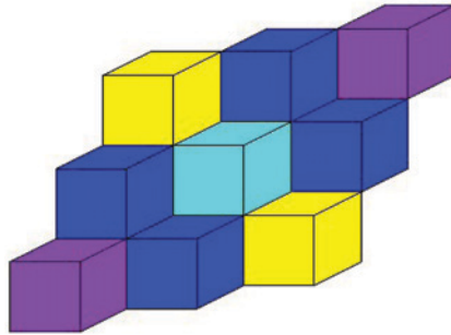
Fig. 7. – La diagonale di una matrice 5 \times 3 \times 3 . Nell'iperdeterminante, che ha grado 30, l'esponente dei coefficienti estremi viola vale 6, per i blu vale 3, per i gialli vale 1 e per il celeste vale 4.
