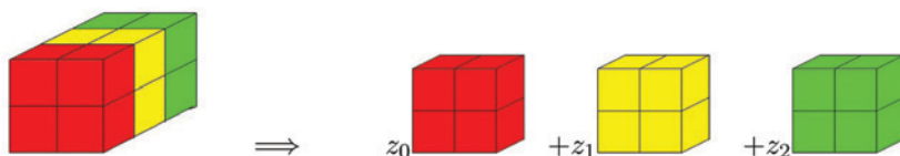
Fig. 9. – Una matrice tridimensionale dà una matrice bidimensionale con coefficienti forme lineari.
