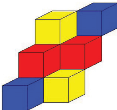
Fig. 6. – La diagonale di una matrice 4 \times 3 \times 2 . Nell'iperdeterminante, che ha grado 12, l'esponente dei coefficienti estremi blu vale 3, per i rossi vale 2 e per i gialli vale 1.
