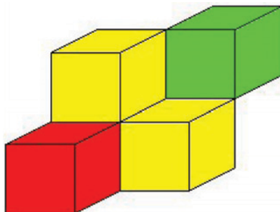
Fig. 5. – La diagonale di una matrice 3 \times 2 \times 2 . Nell'iperdeterminante, che ha grado 6, l'esponente dei coefficienti mediani gialli vale 1, mentre agli estremi vale 2.
