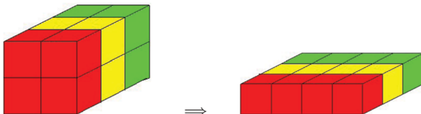
Fig. 2. – Appiattimento di una matrice 3 \times 2 \times 2 su una matrice 3 \times 4
