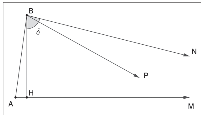
FIGURA 1 – La definizione di parallelismo.
