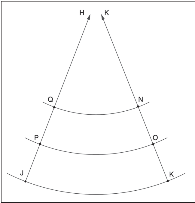
FIGURA 3 – Archi concentrici di L -linee. Posto \widehat{JK}/\widehat{PO} = X e \widehat{JP} = \widehat{OK} = x , si ha X = e^{x/k} .
