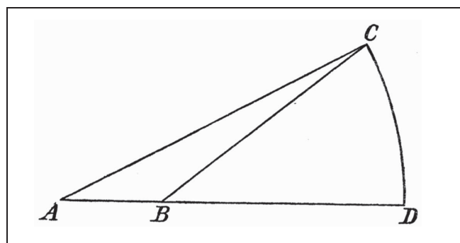
FIGURA 11 – Tratta da [Gauss Werke 1863-1933, VIII, p. 215].
