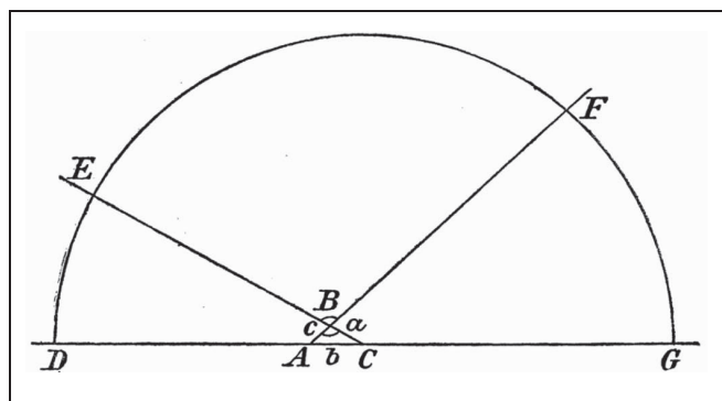
FIGURA 10 – Tratta da [Gauss Werke 1863-1933, VIII, p. 213].
